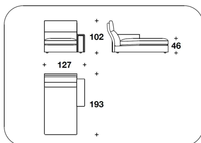
EDE (CLD) - EDE (CLS) CHAISE LONGUE : ALTA DESTRA O SINISTRA / HIGH RIGHT OR LEFT 127x193x102H. - H.S.46cm 50x76x40H. - H.S.18"
