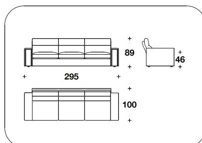
EDE (D4B) DIVANO BASSO 4 POSTI / 4 SEATER LOW SOFA 295x100x89H. - H.S.46cm 116x39 1/3x35H. - H.S.18"
