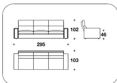
EDE (D4) DIVANO ALTO 4 POSTI / 4 SEATER HIGH SOFA 295x103x102H. - H.S.46cm 116x40 2/3x40H. - H.S.18"
