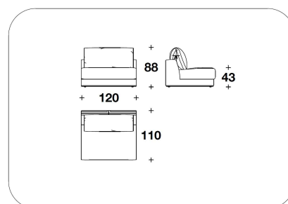
FED (E1CNGT) ELEMENTO SEDUTA SENZA BRACCIOLO / SEAT ELEMENT WITHOUT ARMREST 120x110x88H. - H.S.43 cm 47 1/3x43 1/3x34 2/3H. - H.S.17 "
