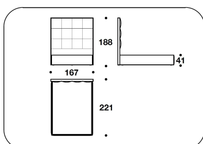
DMN (QUSAI) QUEEN USA : LETTO PER MATERASSO / BED FOR MATTRESS 152x205 - 167x221x188H. - H.B.41 cm 60x80 2/3 - 65 2/3x87x74H. - H.B.16 1/4 "
