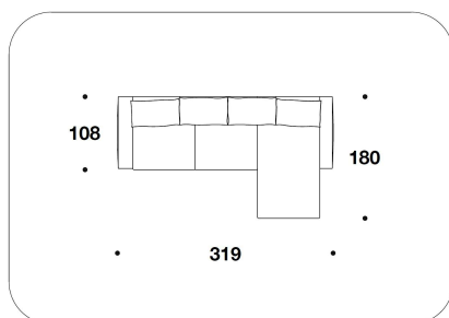
A2E (AND) - A2E (ANS) COMPOSIZIONE / SECTIONAL SOFA 319x108-180x85H. - H.S.45cm 125 2/3x42 2/3-71x33 1/3H. - H.S.17 3/4"
