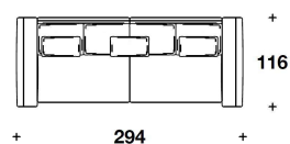
ELN (AE1D) + ELN (AE1S) A) : ESEMPIO DI COMPOSIZIONE / SECTIONAL SOFA EXAMPLE 294x116x98H. - H.S.47 cm 115 2/3x45 2/3x38 2/3H. - H.S.18 2/4 "
