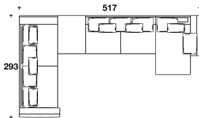
ELN (AD4AS) + ELN (POUR) + ELN (AE2C) + ELN (ACLD) F) : ESEMPIO DI COMPOSIZIONE / SECTIONAL SOFA EXAMPLE 517x293x98H. - H.S.47cm 203 1/2x115 1/3x38 2/3H. - H.S.18 2/4"
