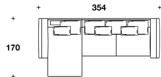
ELN (ACLS) + ELN (AE2D) B) ESEMPIO DI COMPOSIZIONE / SECTIONAL SOFA EXAMPLE 354x170x98H. - H.S.47cm 139 1/2x67x38 2/3H. - H.S.18 2/4"
