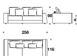
ELN (AD1AD) - ELN (AD1AS) DIVANO ANGOLARE 1 POSTO CON BRACCIOLO DX O SX / 1 SEATER CORNER SOFA WITH RIGHT OR LEFT ARM 256x116x98H. - H.S.47 cm 100 2/3x45 2/3x38 2/3H. - H.S.18 2/4 "
