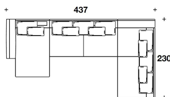
ELN (ACLS) + ELN (AE2C) + ELN (AE1AS) I) ESEMPIO DI COMPOSIZIONE / SECTIONAL SOFA EXAMPLE 437x360x98H. - H.S.47cm 172x141 1/2x38 2/3H. - H.S.18 2/4 "
