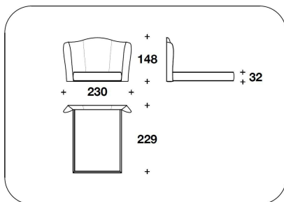
JOL (QUSA) QUEEN USA : LETTO PER MATERASSO / BED FOR MATTRESS 152x205 - 230x229x148H. - H.B.32cm 60x80 2/3 - 90 2/3x90x58 1/3H. - H.B.12 2/4"
