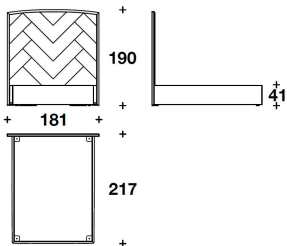
CVR (QUSAE) - CVR (QUSAL) QUEEN USA : LETTO PER MATERASSO / BED FOR MATTRESS 152x205 - 181x217x190H. - H.B.41cm 60x80 2/3 - 71 1/3x85 1/3x74 2/3H. - H.B.16 1/4"
