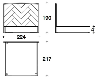
CVR (KUSAE) - CVR (KUSAL) KING USA : LETTO PER MATERASSO / BED FOR MATTRESS 195x205 - 224x217x190H.-H.B.41cm 76 2/3x80 2/3 - 88 1/3x85 1/3x74 2/3H.- H.B.16 1/4"
